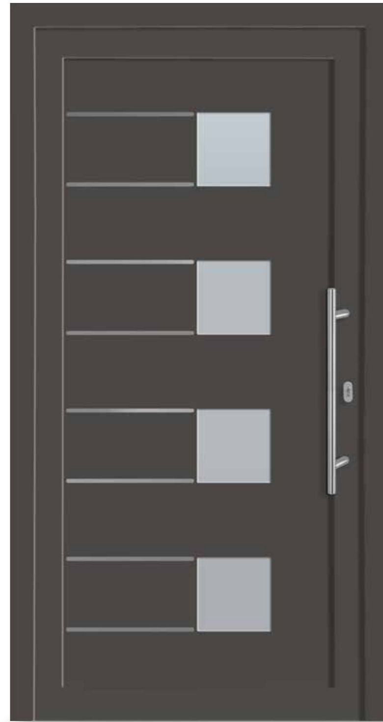
M-230 Ansicht A / DIN rechts Applikationen in Edelstahloptik außen und Rahmen in Edelstahloptik innen ■ Dekor Eisenglimmer ■ Isolierglas Satinato weiß | GG 2 ■ Griff ZAE 6s, 600 mm | PG 6
